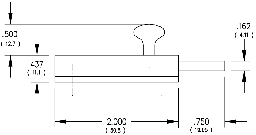
5204 RIM BOLT
